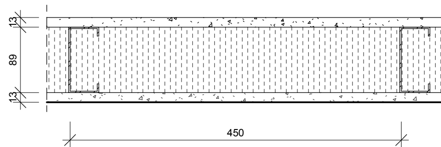
Standard skillevægge:
