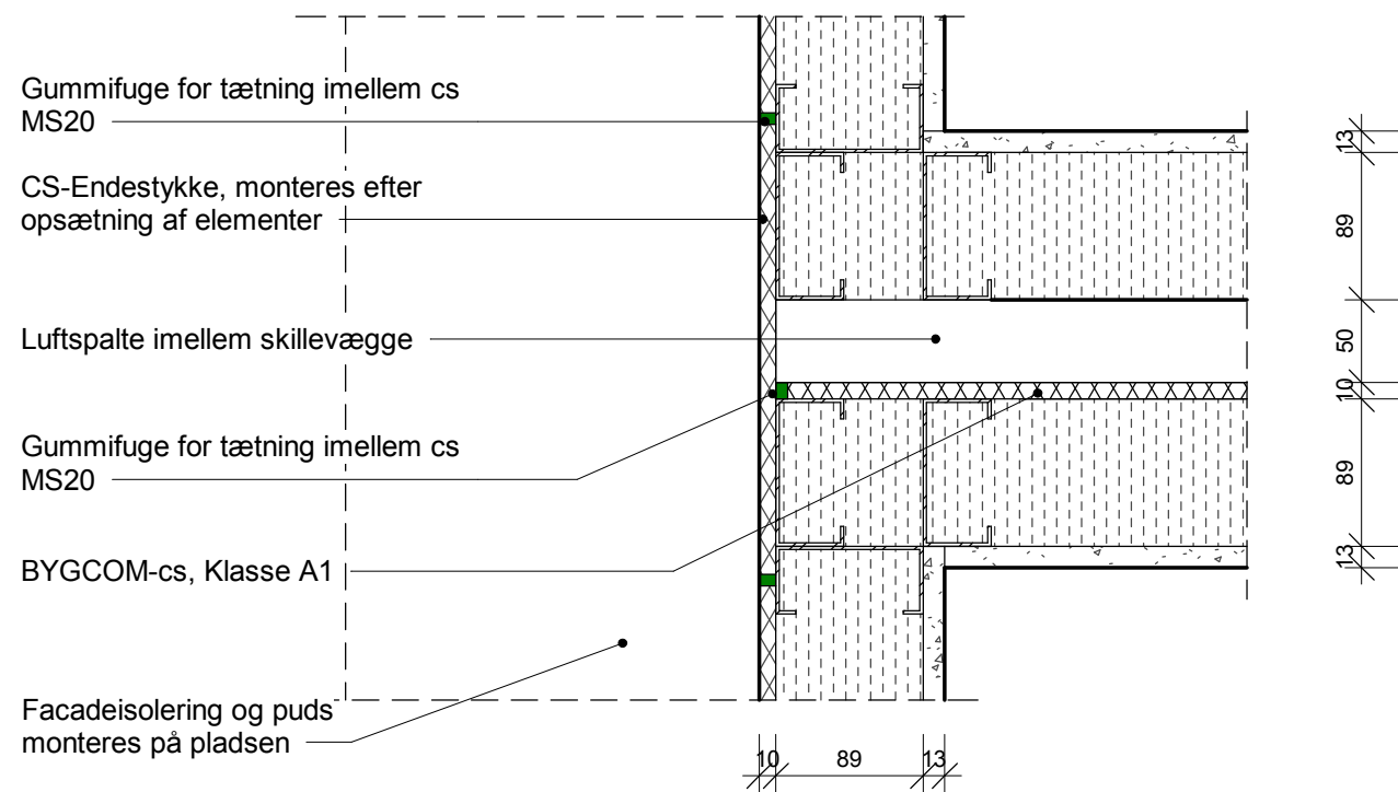
Standart lejlighedsskel (Plan)
