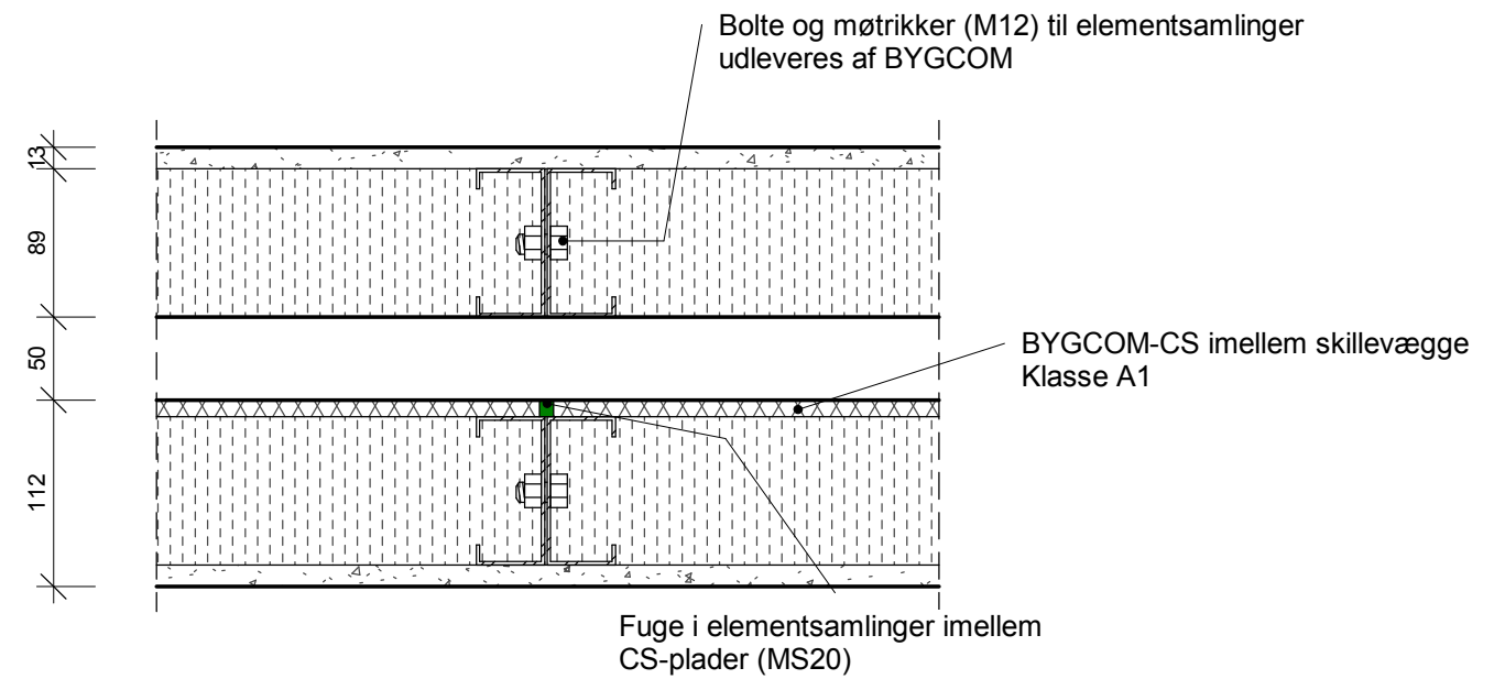
Lejlighedsskel (Plane):
